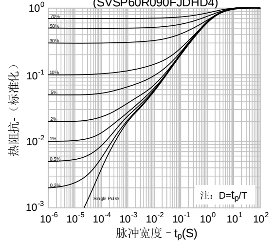
图16-3.瞬态热阻抗 vs. 脉冲宽度 (SVSP60R090FJDHD4)
