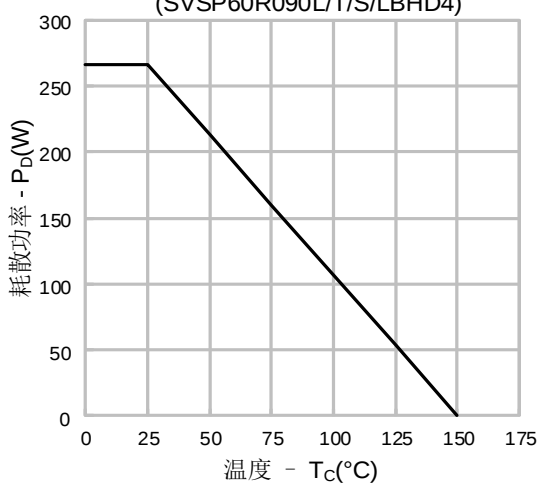
图14-2. 耗散功率vs.温度 (SVSP60R090L/T/S/LBHD4)
