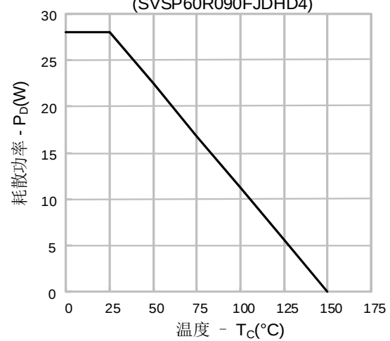
图14-3. 耗散功率vs.温度 (SVSP60R090FJDHD4)
