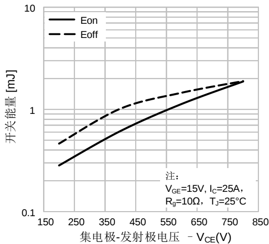
图 29. 开关损耗vs.集电极-发射极电压
