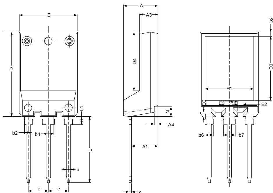
TO-247PH-3L
