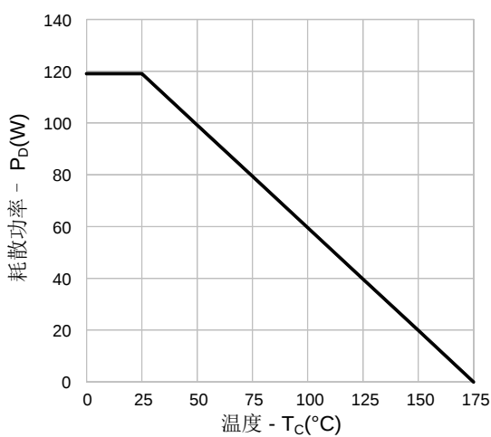
图 17. 耗散功率 vs. 温度
