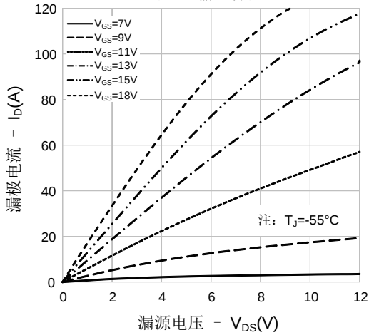
图 3. 输出特性
