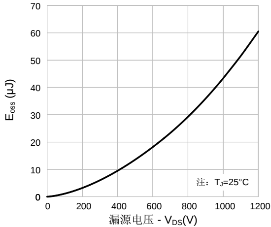
图15. 电容特性
