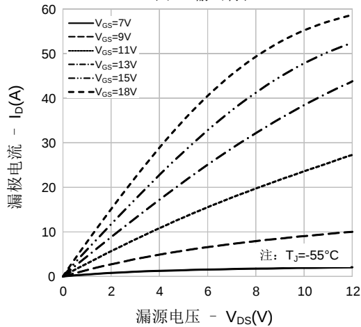
图 3. 输出特性
