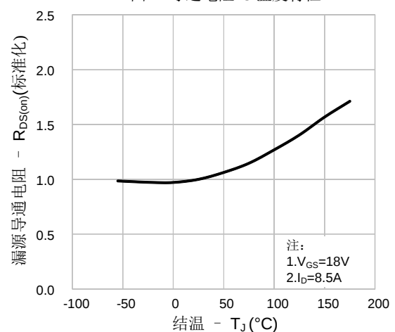
图 4. 导通电阻vs.温度特性
