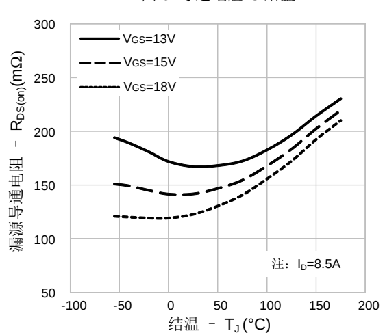
图 6. 导通电阻vs.结温
