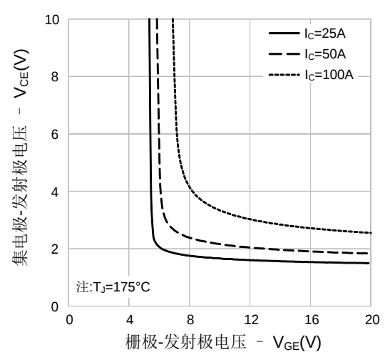
图6. 饱和电压VS. Vge
