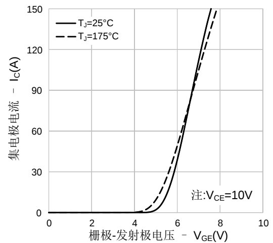
图4. 传输特性
