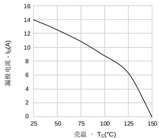
图10. 最大漏极电流vs. 壳温
