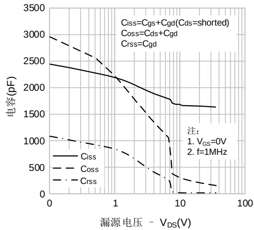
图5. 电容特性
