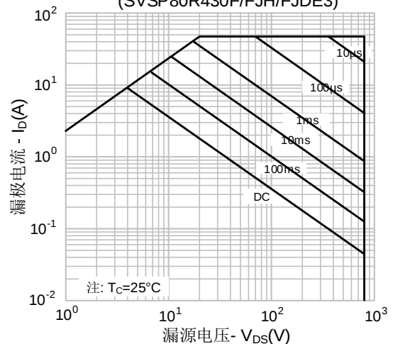
图 12-1. 最大安全工作区域 (SVSP80R430F/FJH/FJDE3)
