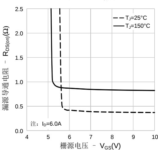
图 5. 导通电阻vs.栅源电压
