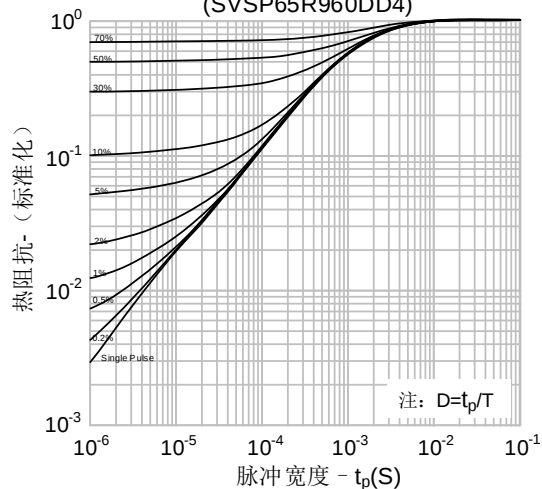
图16-1.瞬态热阻抗 vs. 脉冲宽度 (SVSP65R960DD4)
