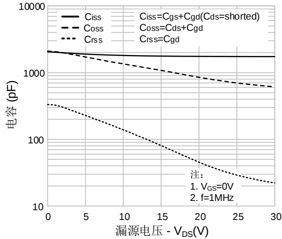
图7. 电容特性
