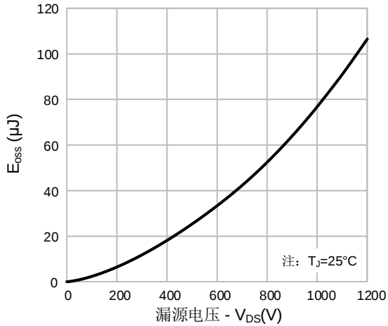
图15. 电容特性
