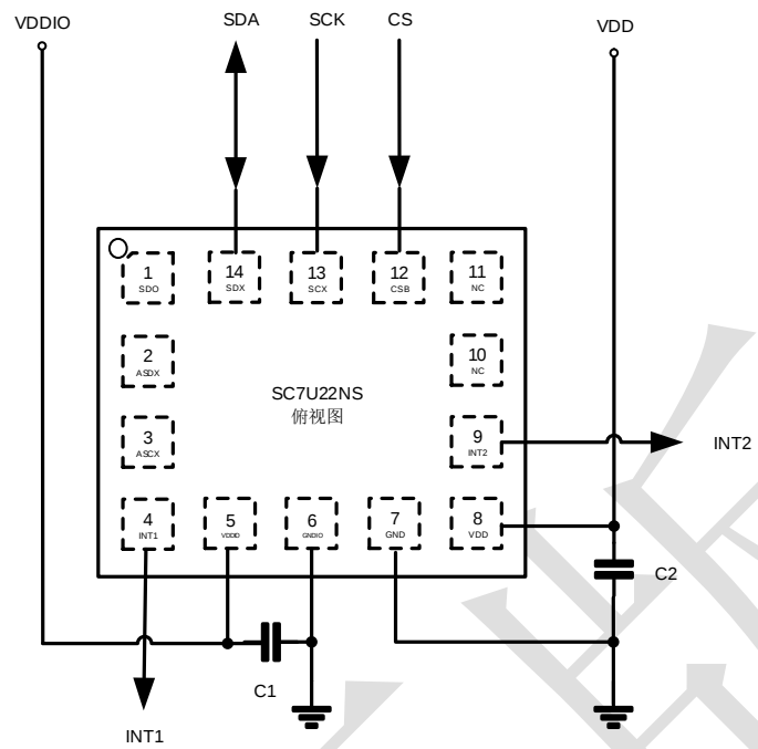
3线SPI通信方式连接原理图
