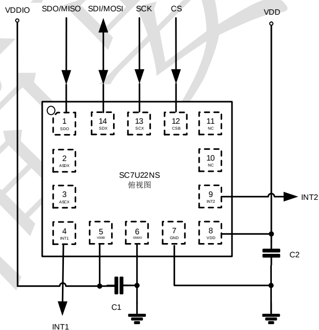
4线SPI通信方式连接原理图
