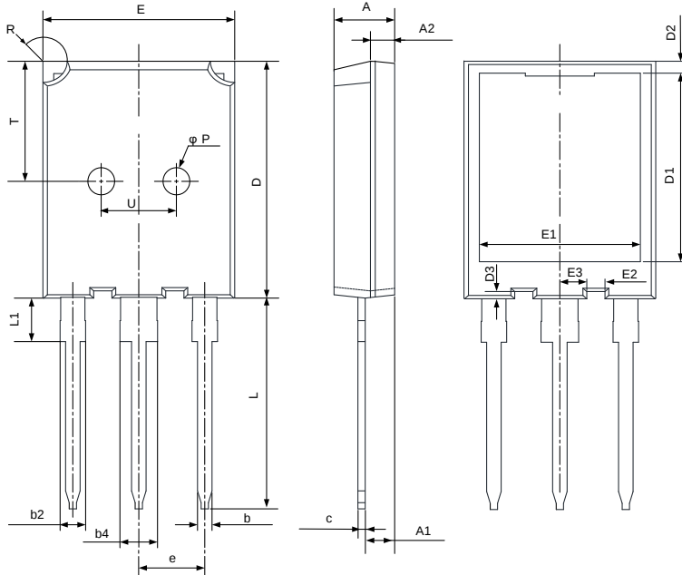
TO-247P-3L
