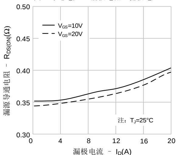
图3. 导通电阻vs.漏极电流、栅极电压
