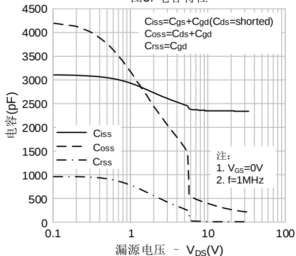
图5. 电容特性
