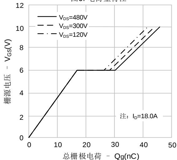
图6. 电荷量特性
