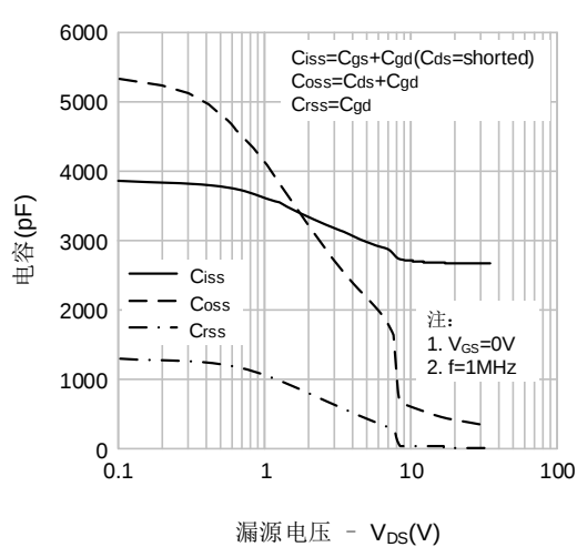
图5. 电容特性
