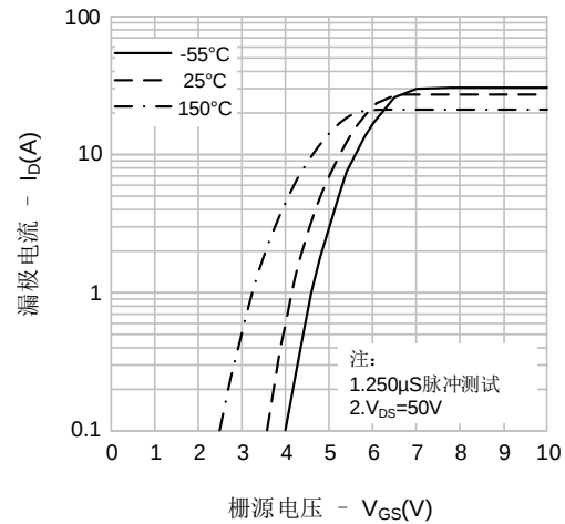
图2. 传输特性
