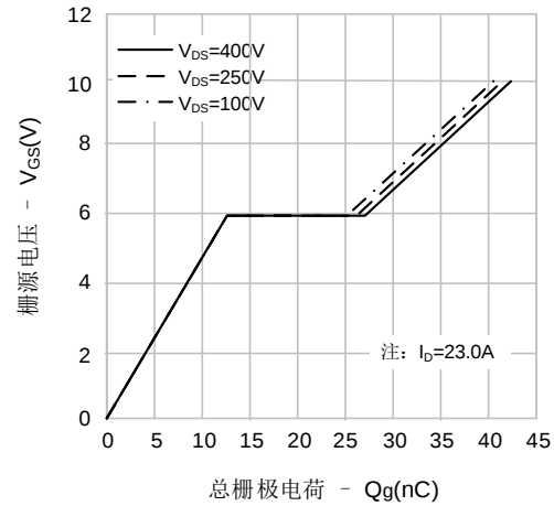
图6. 电荷量特性
