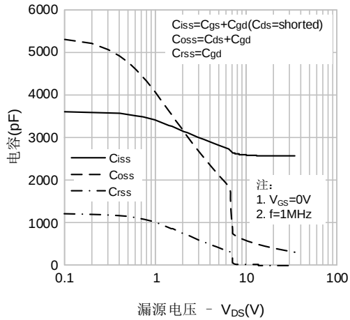
图5. 电容特性
