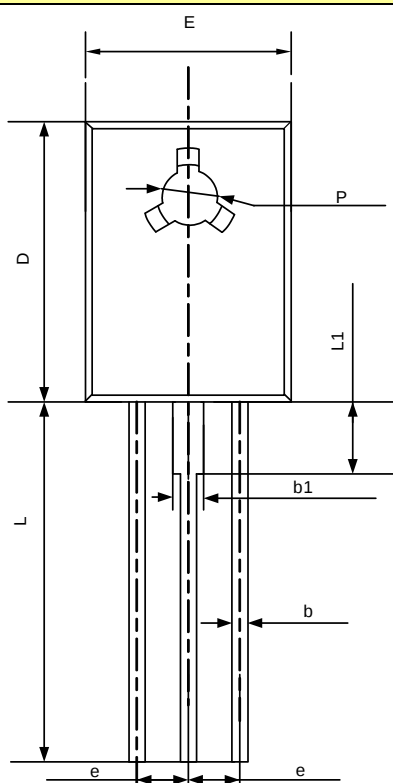
TO-126-3L
