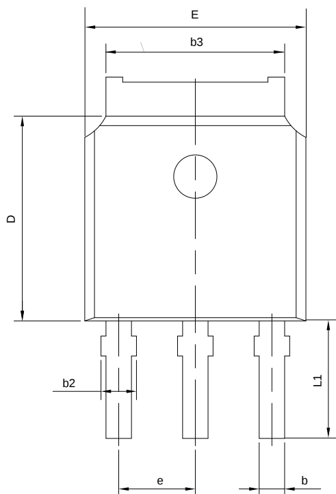
TO-126-3L
