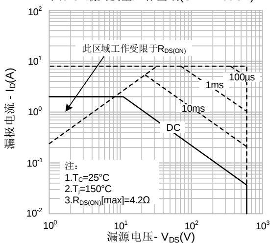
图9-3. 最大安全工作区域(SVF2N60CF)
