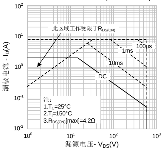
图9-3. 最大安全工作区域(SVF2N60CF)
