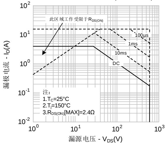
图9-3. 最大安全工作区域(SVF4N60T)
