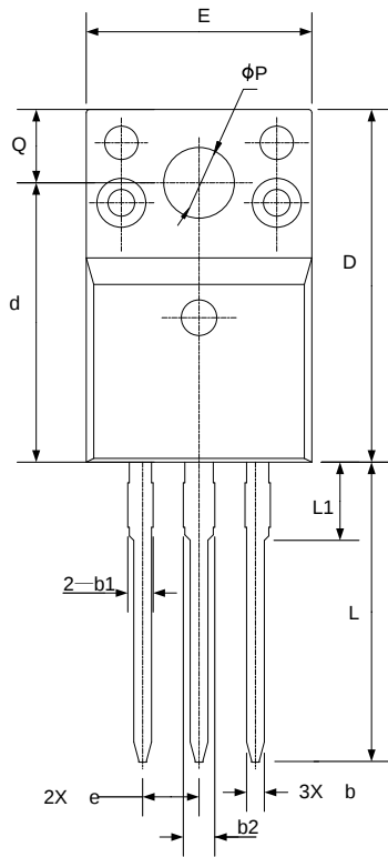
TO-220FQ-3L
