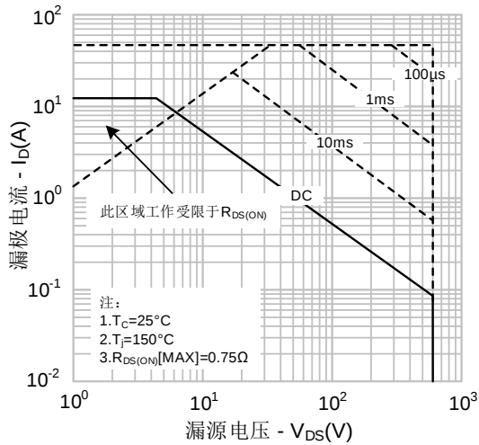
图9-3. 最大安全工作区域(SVF12N60K)
