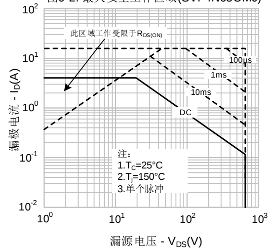
图9-2. 最大安全工作区域(SVF4N65CMJ)
