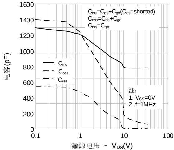
图 5. 电容特性
