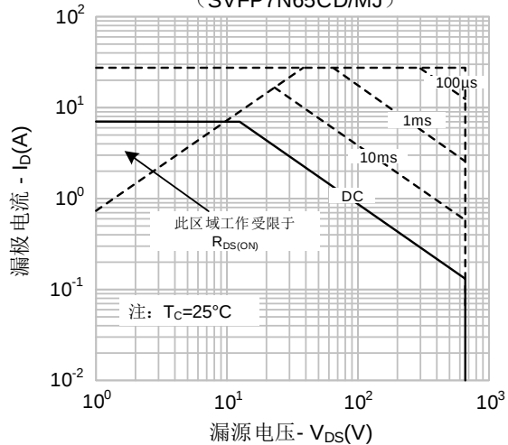
图9. 最大安全工作区域 (SVFP7N65CD/MJ)
