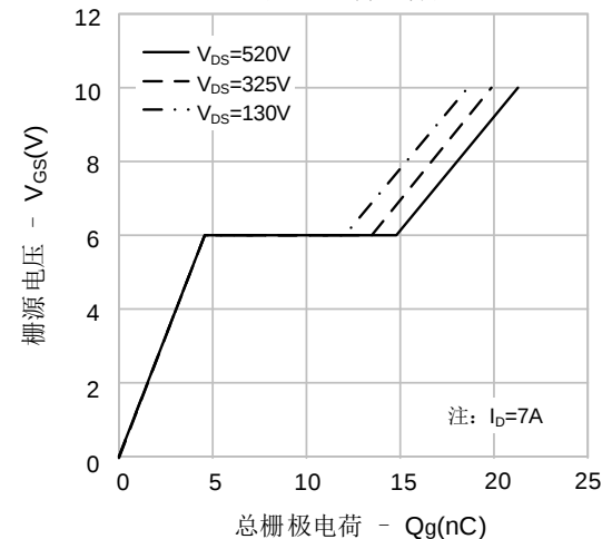
图 6. 电荷量特性
