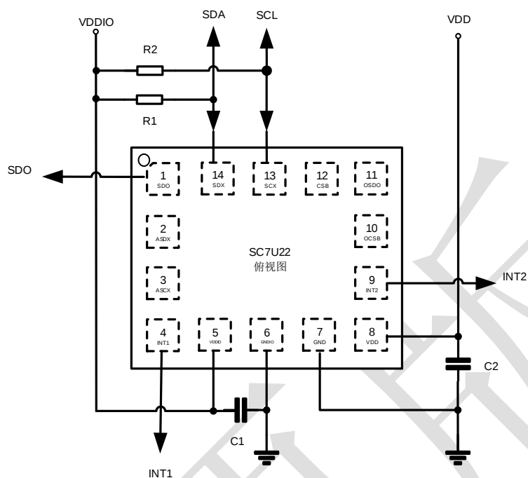
IIC通信方式连接原理图
