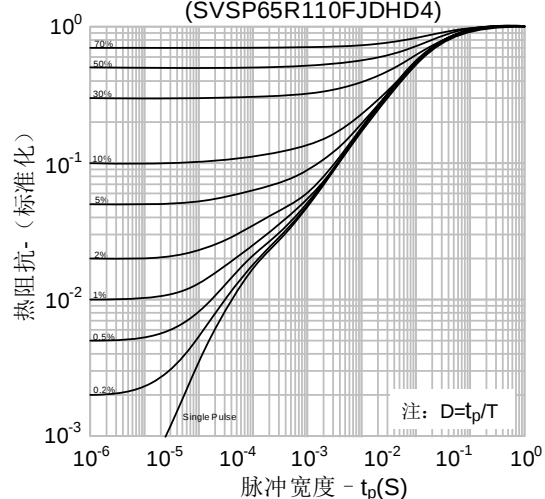
图16-3.瞬态热阻抗 vs. 脉冲宽度 (SVSP65R110FJDHD4)
