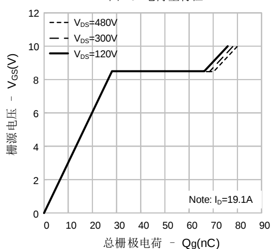
图 10. 电荷量特性
