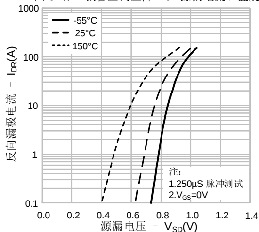
图 8. 体二极管正向压降 vs. 源极电流、温度
