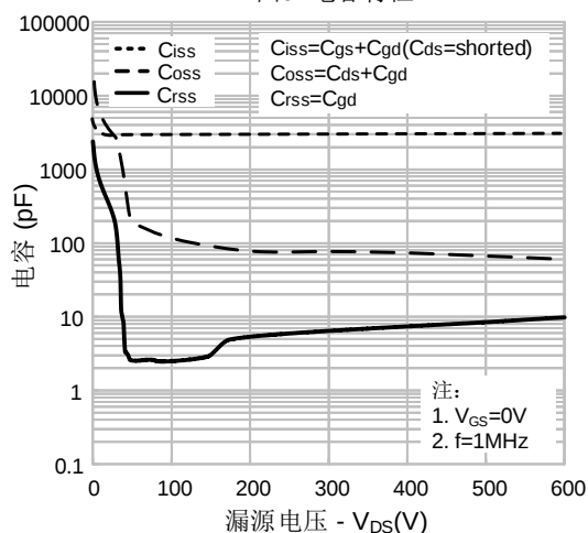
图9. 电容特性
