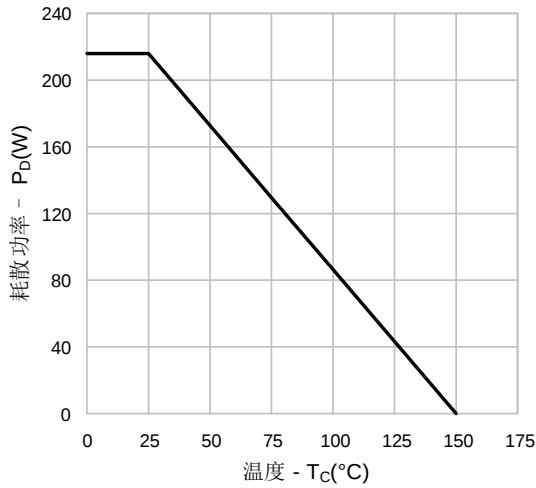
图 12-1. 耗散功率 vs. 温度(SVGP103R1NT)
