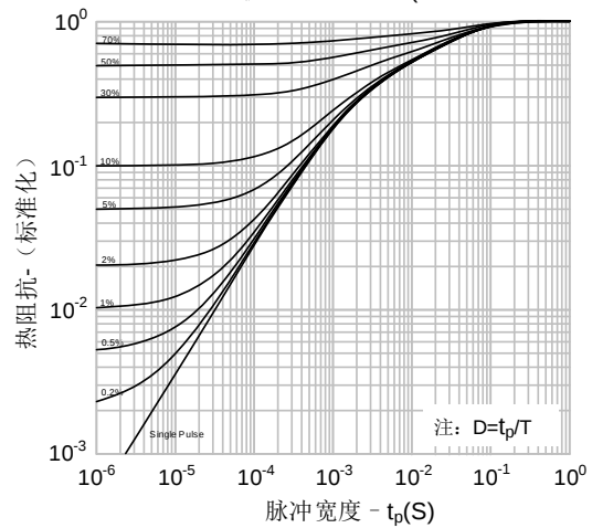
图14-2. 瞬态热阻抗 vs. 脉冲宽度(SVGP103R1NP7)
