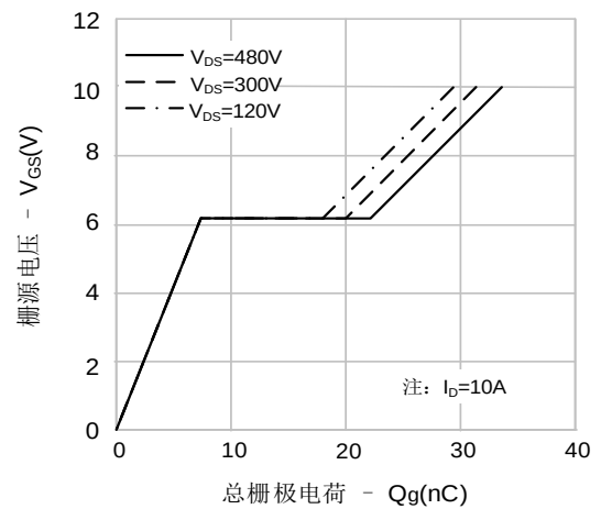
图6. 电荷量特性
