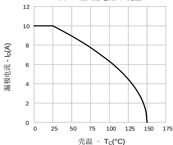
图10. 最大漏电流vs. 壳温
