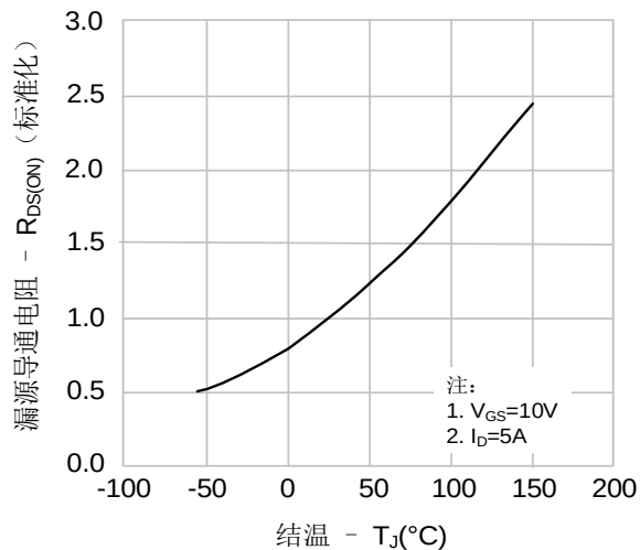
图8. 导通电阻vs.温度特性
