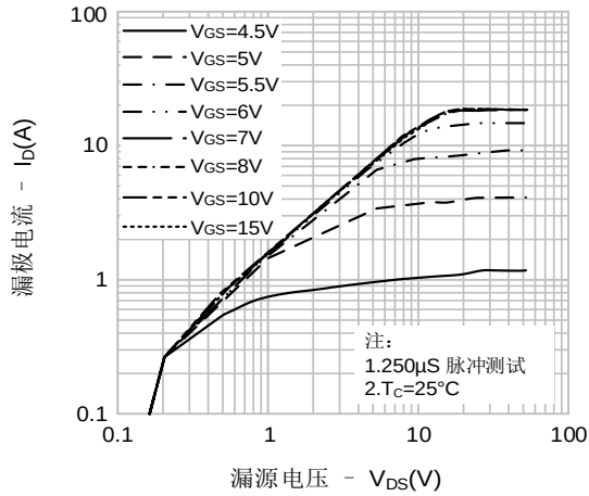
图1. 输出特性
