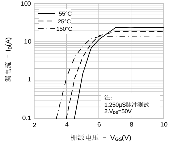
图2. 传输特性
