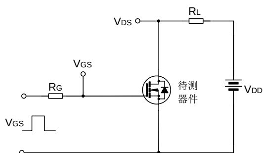
开关时间测试电路及波形图
