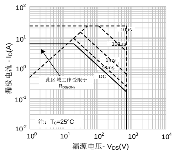
图 12-1. 最大安全工作区域 (SVF7N70AD/MJ)
