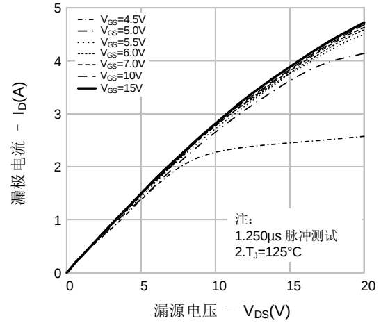
图 2. 输出特性
