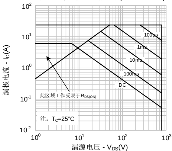
图9-3. 最大安全工作区域(SVF6N80AF)
