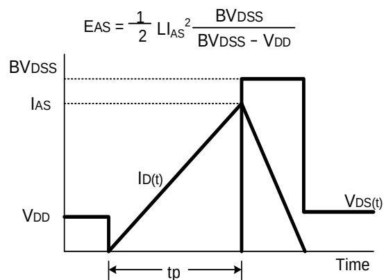
EAS测试电路及波形图
