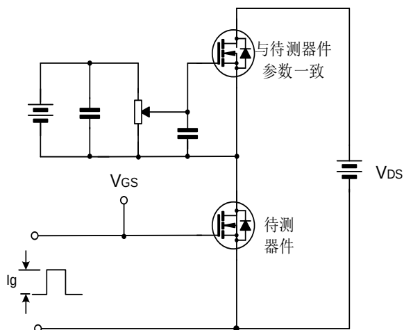
栅极电荷量测试电路及波形图
