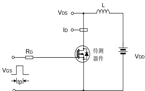
EAS测试电路及波形图
