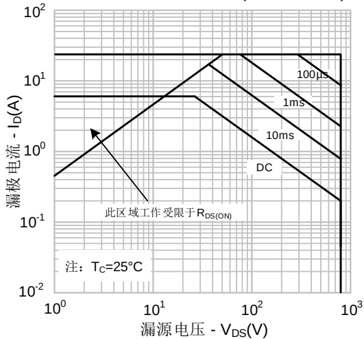
图9-3. 最大安全工作区域(SVF6N80AF)
