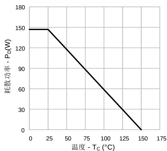
图 13-3. 耗散功率VS.温度(STS65R280SS2)
