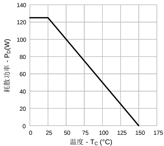
图 13-3. 耗散功率VS.温度(STS65R280SS2)
