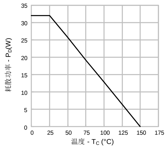
图 13-2. 耗散功率VS.温度(STS65R280FS2)
