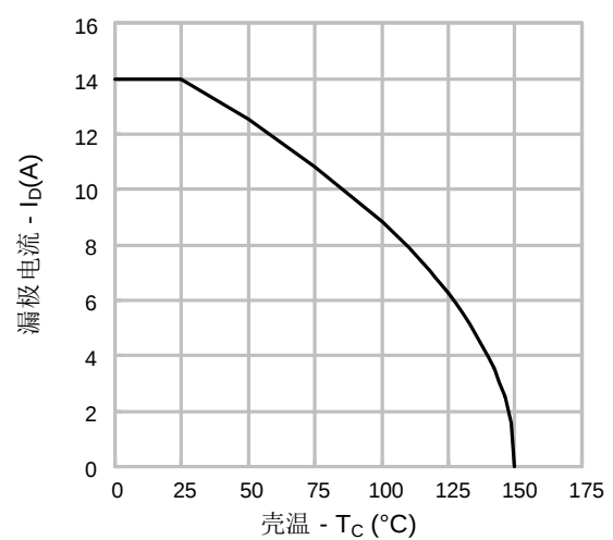
图 14. 漏极电流VS.壳温
