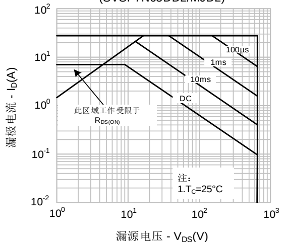
图9-1. 最大安全工作区域 (SVSP7N65DD2/MJD2)
