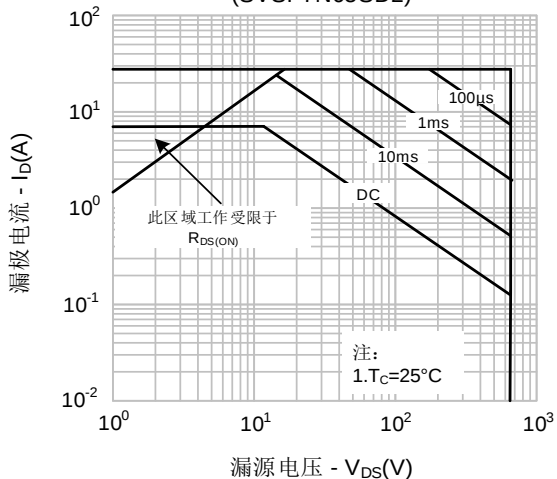
图9-3. 最大安全工作区域 (SVSP7N65SD2)
