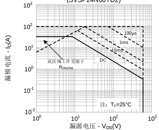
图9-2. 最大安全工作区域 (SVSP24N60TD2)
