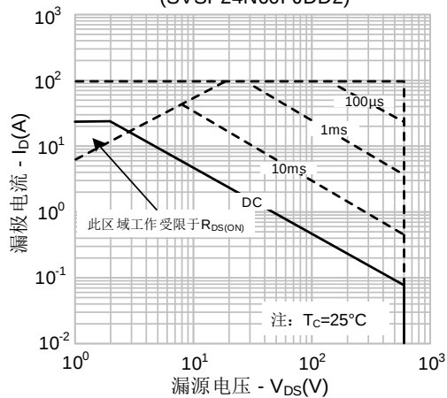
图9-1. 最大安全工作区域 (SVSP24N60FJDD2)
