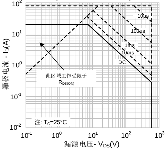
图 13-5. 最大安全工作区域 (SVS60R190P7/PND4)
