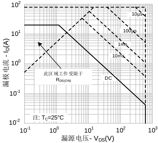
图 13-3. 最大安全工作区域(SVS60R190L8AD4)
