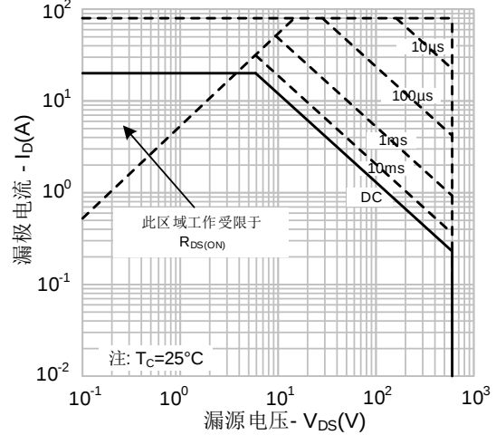
图 13-4. 最大安全工作区域 (SVS60R190T/S/KD4)
