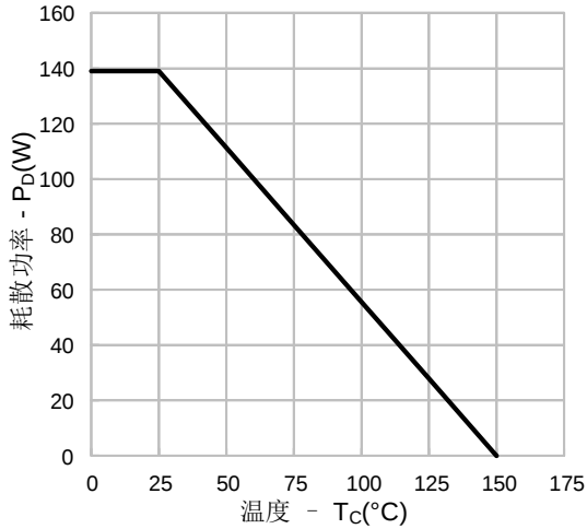
图14-4. 耗散功率vs.温度(SVS60R190T/S/KD4)
