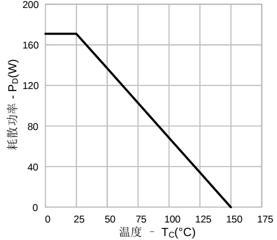
图14-5. 耗散功率vs.温度(SVS60R190P7/PND4)
