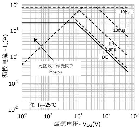
图 13-5. 最大安全工作区域 (SVS60R190P7/PND4)
