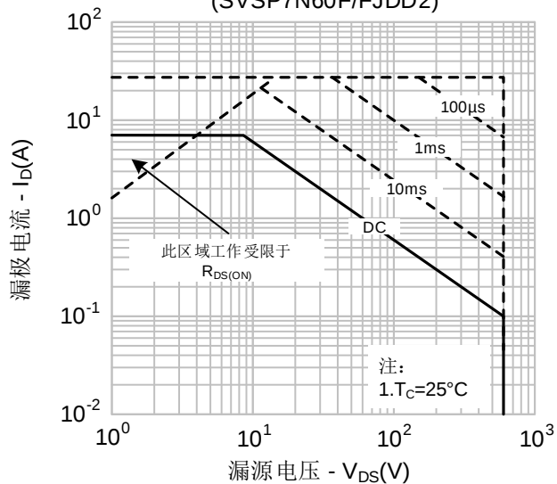
图9-1. 最大安全工作区域 (SVSP7N60F/FJDD2)
