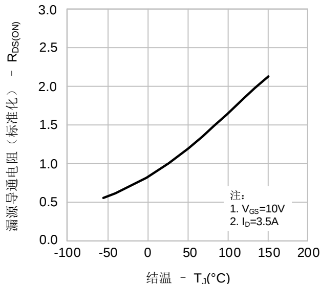
图8. 导通电阻 vs. 温度特性
