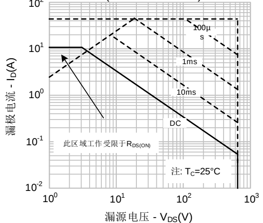
图9.2. 最大安全工作区域 (SVS11N65F/FJD2)
