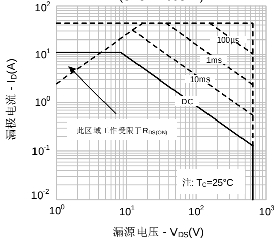
图9.3. 最大安全工作区域 (SVS11N65SD2)
