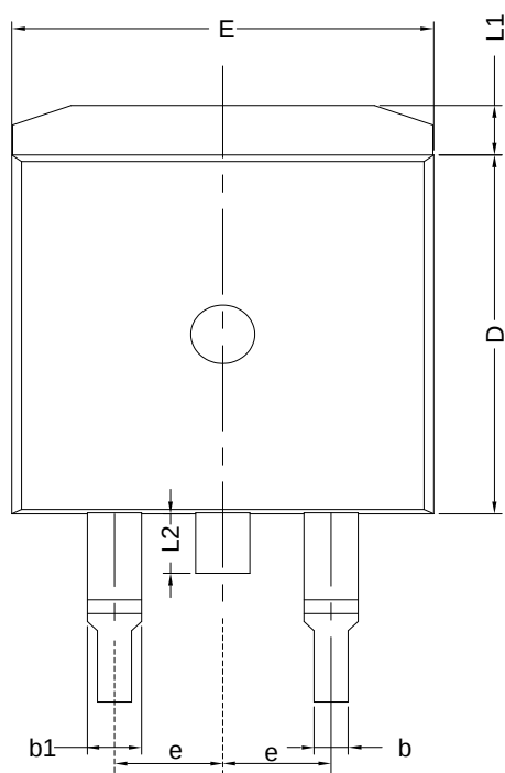
TO-263-2L
