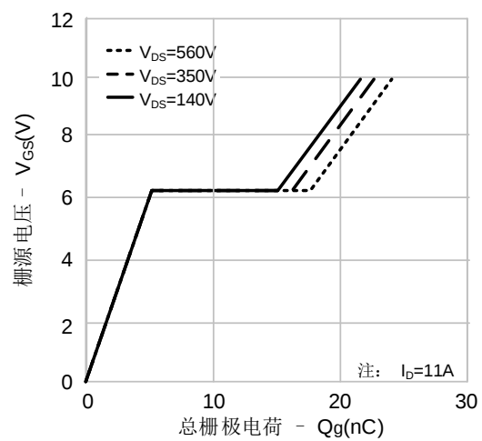
图 6. 电荷量特性
