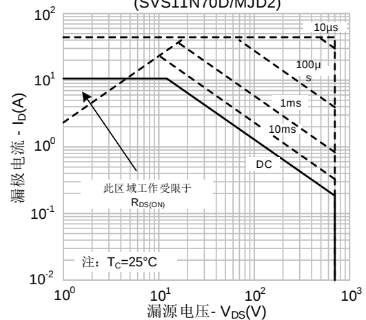
图 9-2. 最大安全工作区域 (SVS11N70D/MJD2)
