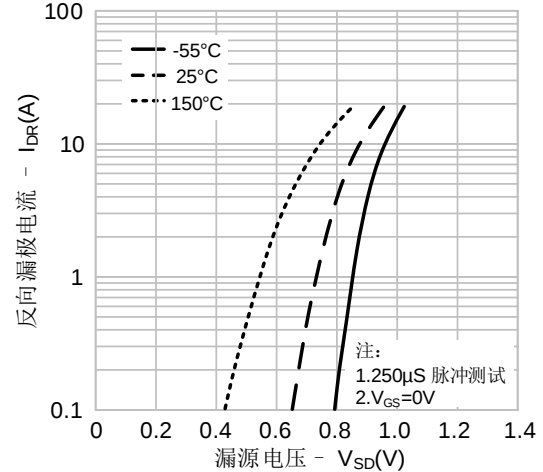
图 4. 体二极管压降 vs. 源极电流、温度
