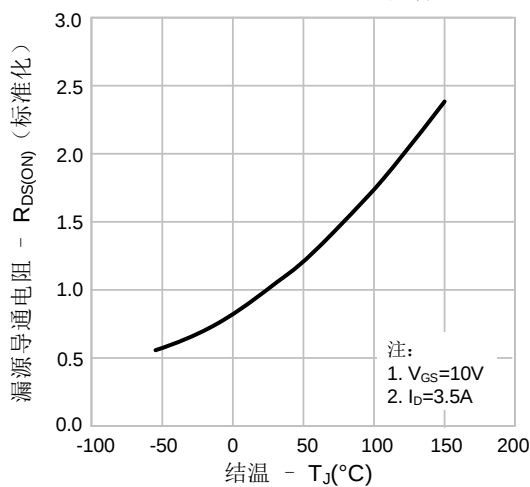
图 11. 导通电阻 vs. 温度特性
