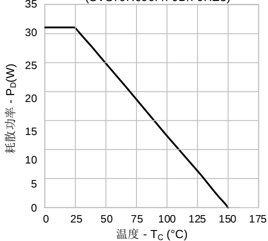
图 13-3. 耗散功率 vs. 温度 (SVS70R600F/FJD/FJHE3)
