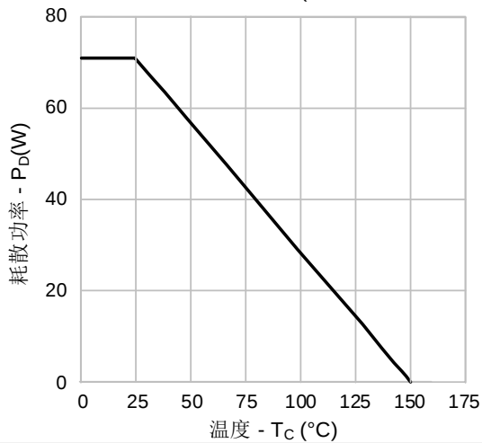
图 13-3. 耗散功率 vs. 温度 (SVS70R600F/FJD/FJHE3)
