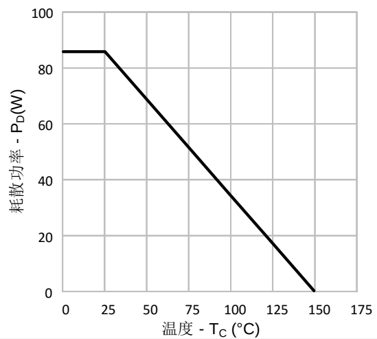
图 13-2. 耗散功率 vs. 温度(SVS70R600SE3)
