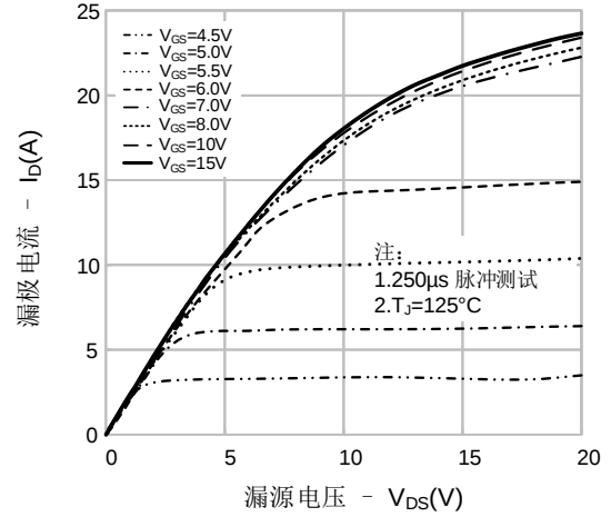
图 2. 输出特性
