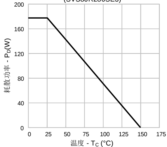
图 13-2. 耗散功率 vs. 温度 (SVS80R280SE3)
