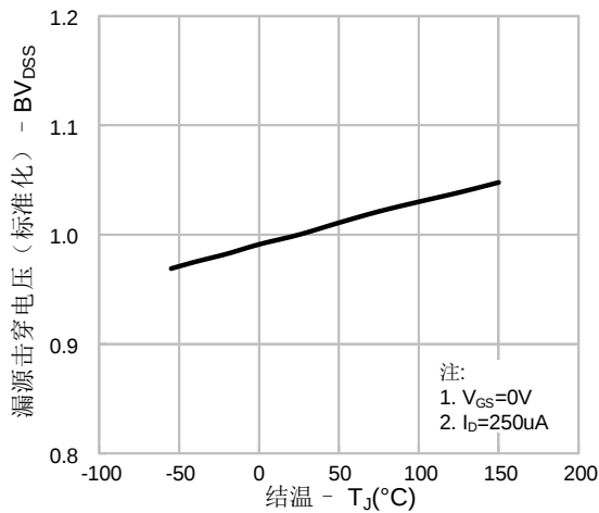
图 9. 击穿电压 vs. 温度
