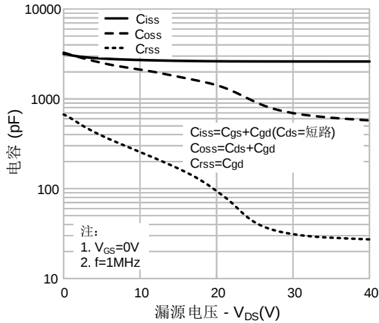
图 7. 电容特性
