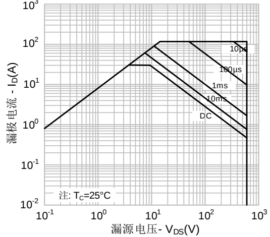
图 13-4. 最大安全工作区域(SVSP60R125KD4)
