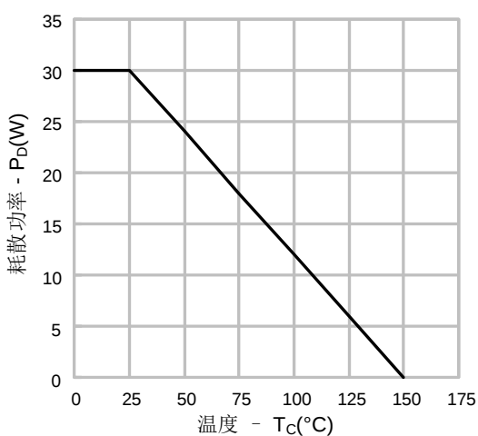
图14-1. 耗散功率vs.温度(SVSP60R125FJDD4)
