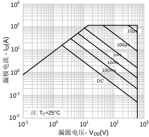
图13-3. 最大安全工作区域(SVSP60R125L8AD4)
