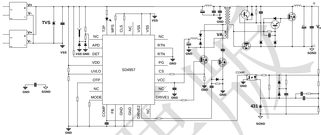
有源钳位正激同步整流方案典型应用图
