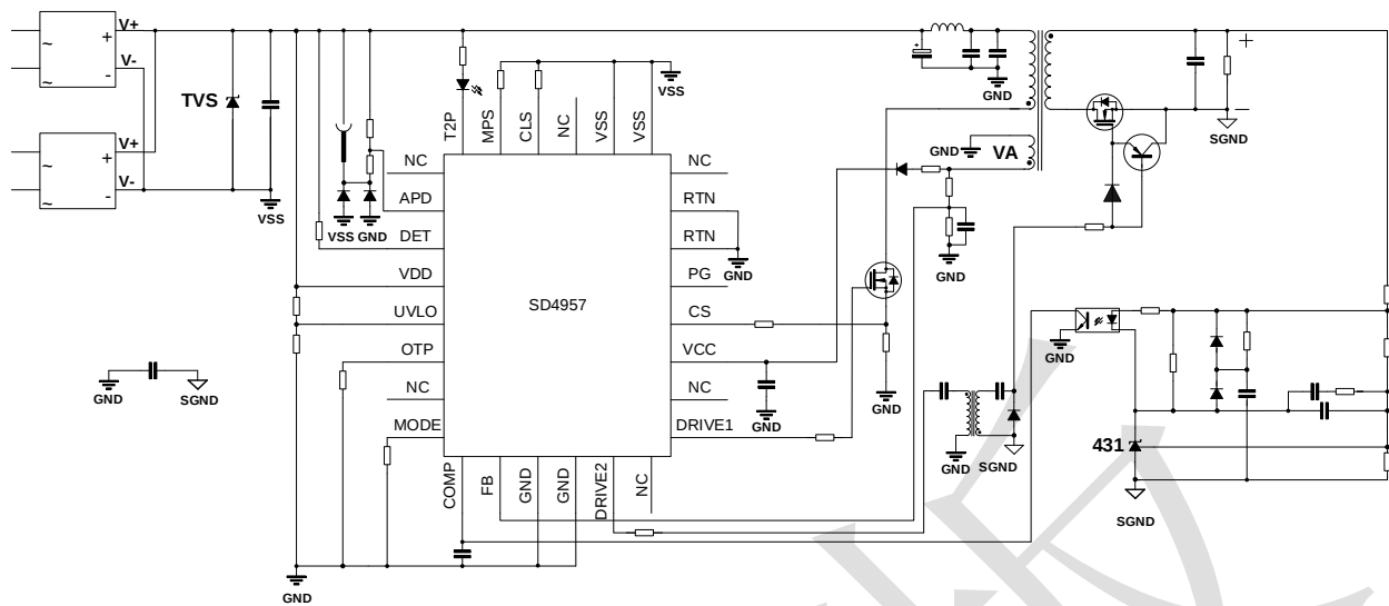
SSR反激同步整流方案典型原理图
