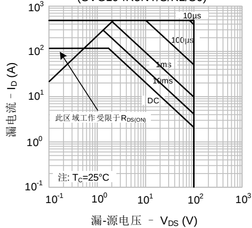
图 9-1. 最大安全工作区域 (SVG104R5NT/S/KL/S6)
