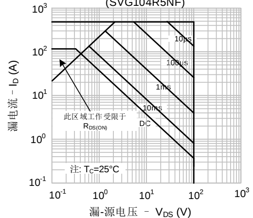
图 9-2. 最大安全工作区域 (SVG104R5NF)
