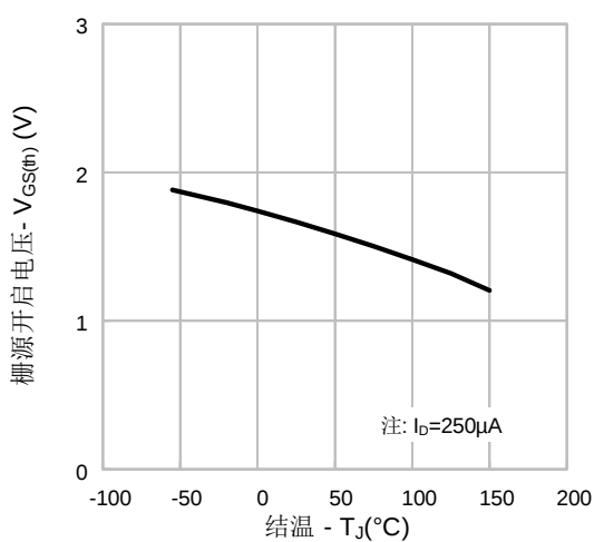
图 5. 开启电压 vs. 温度
