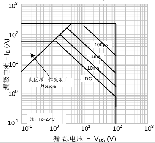
图 11-2. 最大安全工作区域(SVG10170NT)
