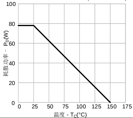
图 12-2. 耗散功率 vs. 温度(SVG10170NT)
