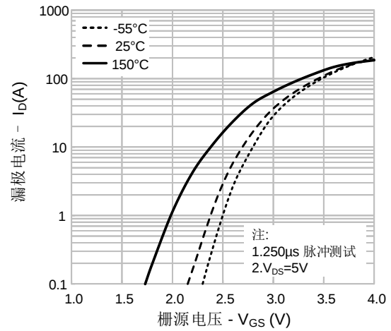
图 2. 传输特性
