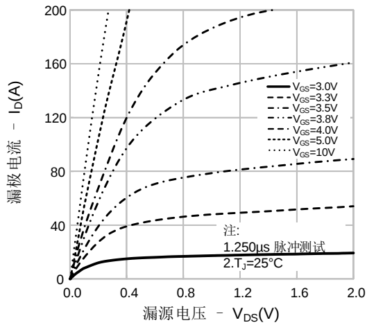
图 1. 输出特性
