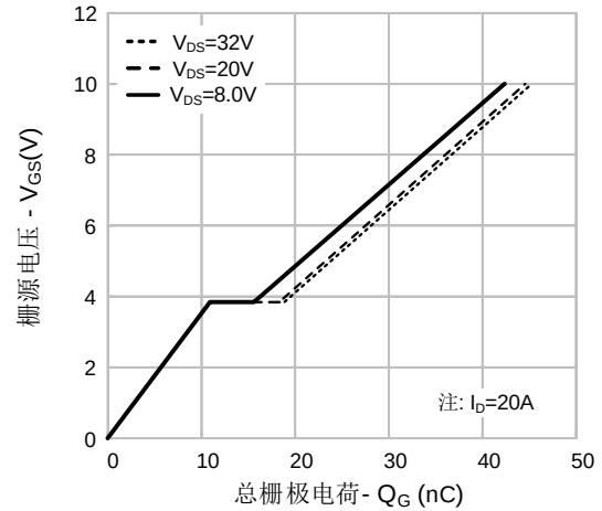
图 8. 电荷量特性
