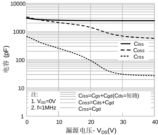
图 7. 电容特性
