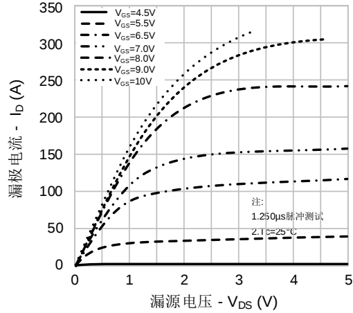
图 1. 输出特性
