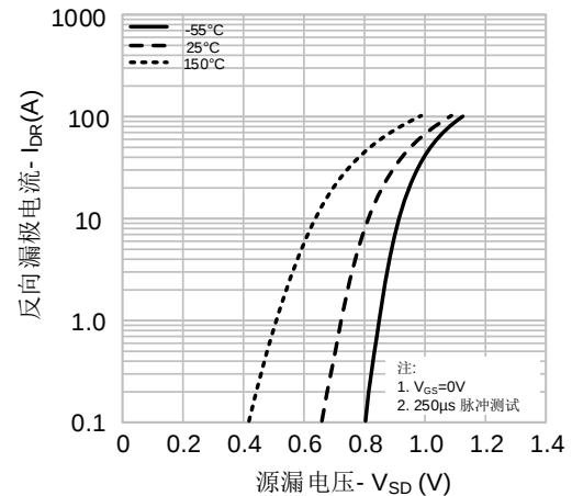
图 4. 体二极管正向压降 vs. 源极电流和温度
