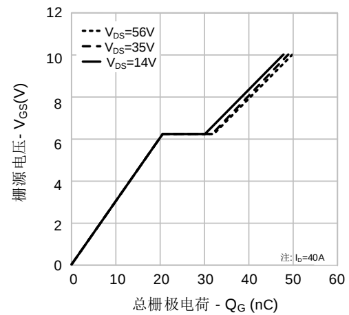
图 6. 电荷量特性
