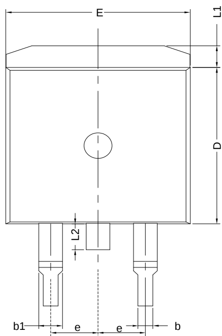
TO-263-2L
