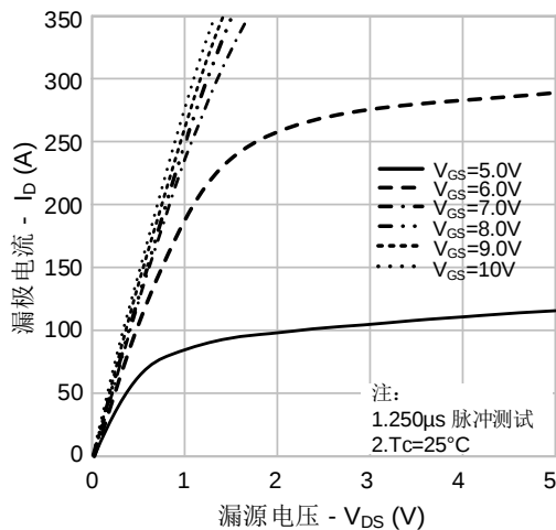
图 1. 输出特性
