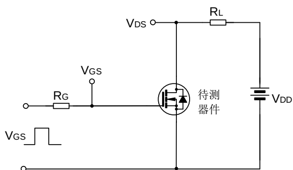
开关时间测试电路及波形图
