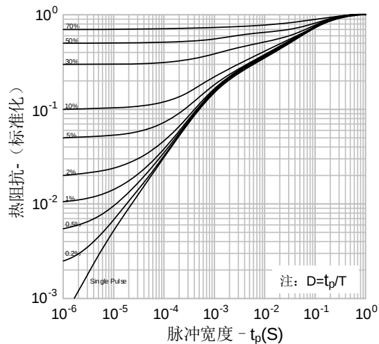
图16.瞬态热阻抗 vs. 脉冲宽度
